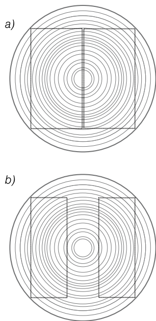
Obrázok 1: Rezanie polením (a) s polením s vyrezaním jadrovej fošne (b)
