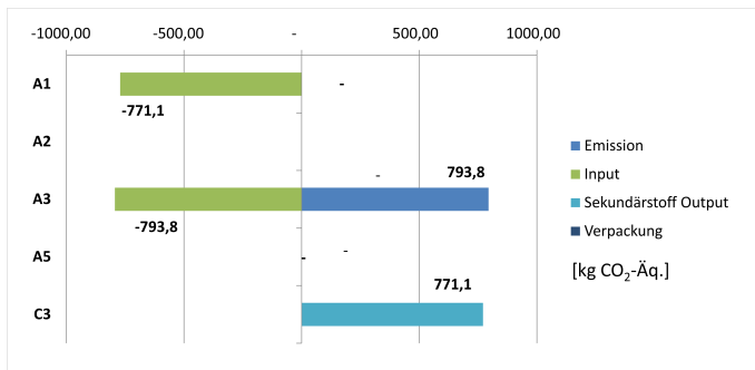
Abb.2: Holzhäufige CO 2 -Produktsystemein- und -ausgänge. Die inverse Vorzeichengebung der In- und Outputs trägt der ökobilanziellen CO 2 -Flussbetrachtung aus Sicht der Atmosphäre Rechnung.
